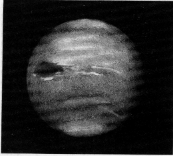
नेपच्यूनचा पृष्ठभाग व त्यावरील चक्रीवादळ (द ग्रेट डार्क स्पॉट)
